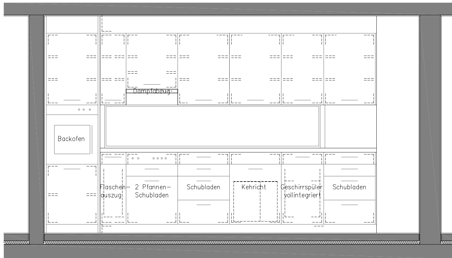
ANSICHT A
