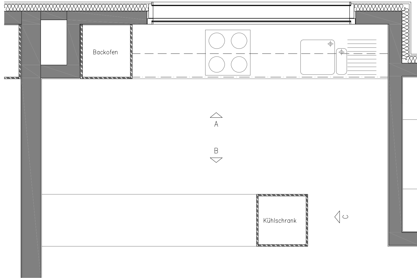
GRUNDRISS
