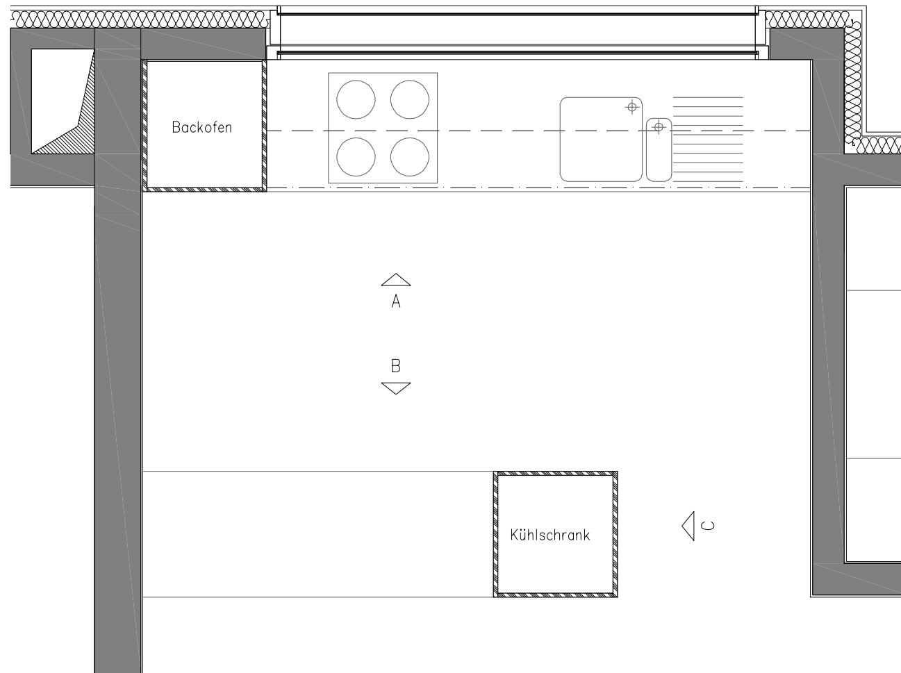
GRUNDRISS
