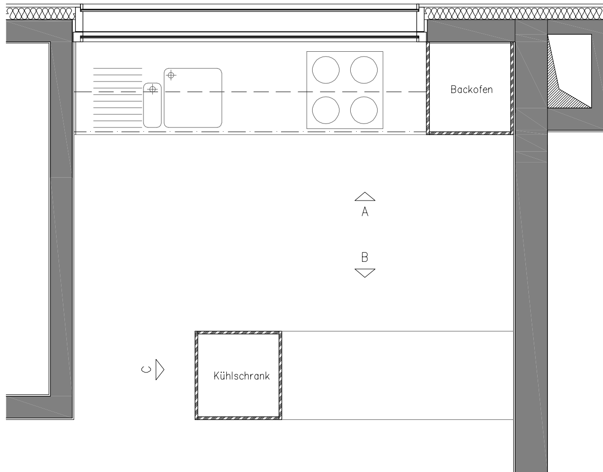
GRUNDRISS
