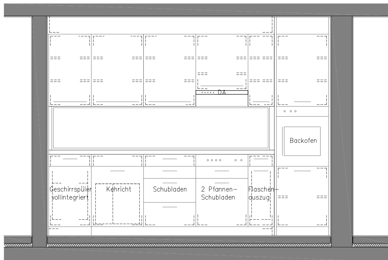
ANSICHT A
