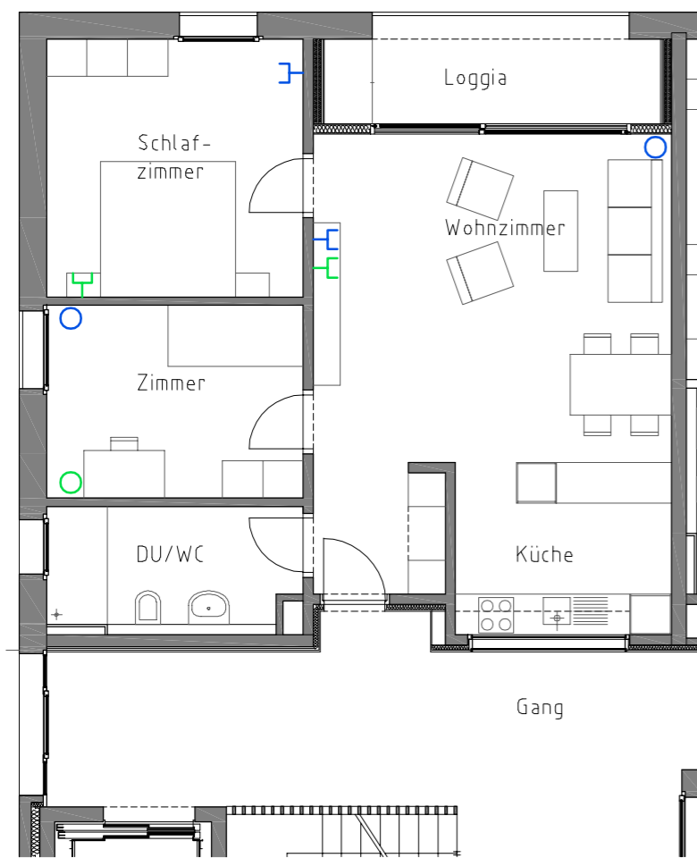
WOHNUNG TYP 5
