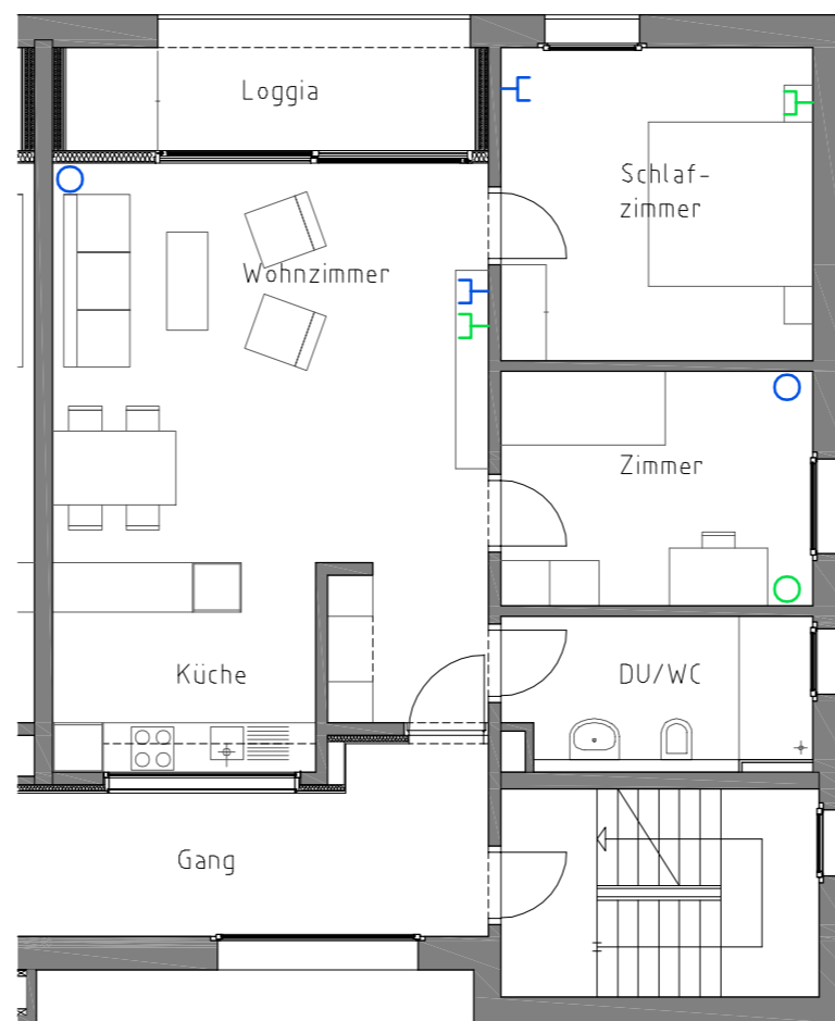
WOHNUNG TYP 6
