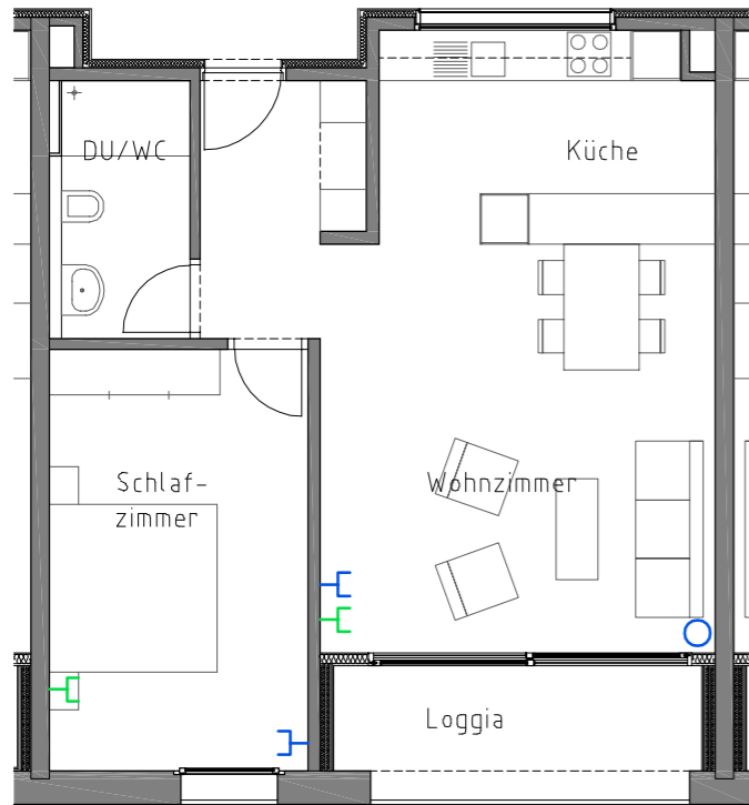
WOHNUNG TYP 3
