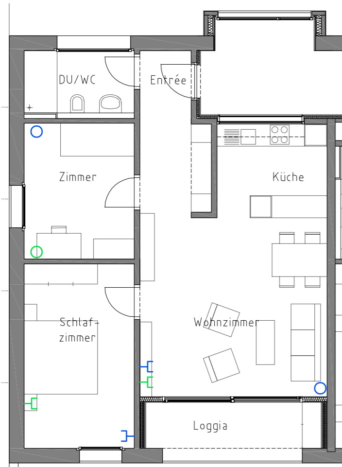
WOHNUNG TYP 1
