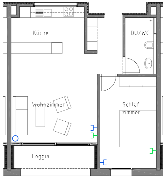
WOHNUNG TYP 4
