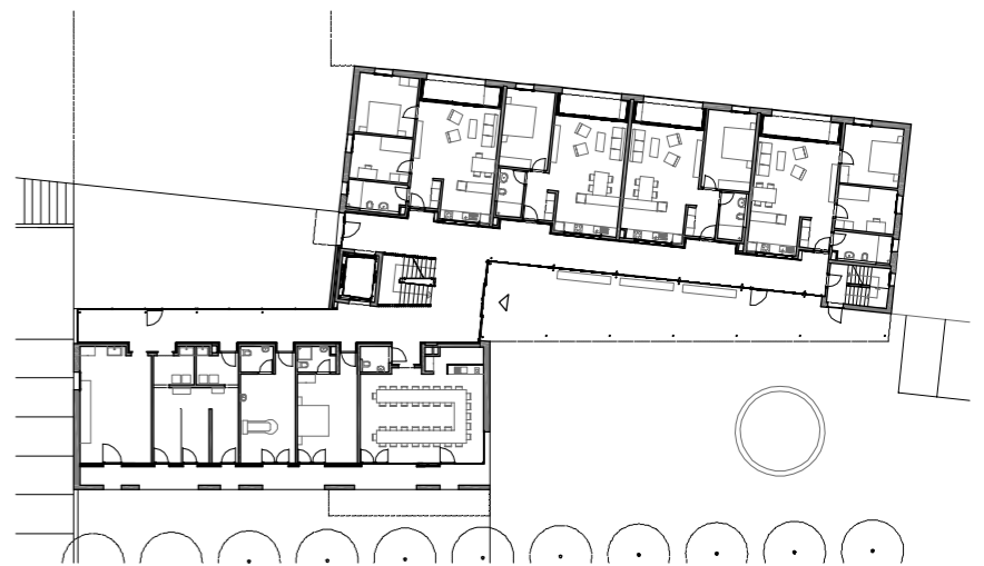
ERDGESCHOSS
